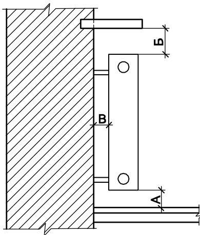
А, Б, В — расстояния от отопительного прибора до строительных конструкций
